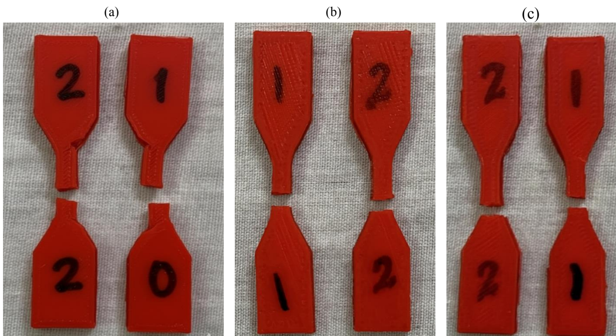
Fig. 14. Raster angles.
