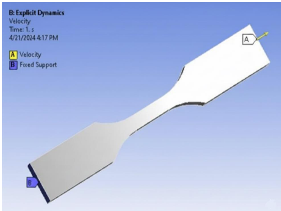
Fig. 8. ANSYS mechanical.
