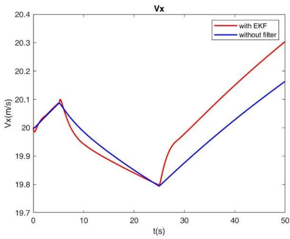
a. longitudinal speed
